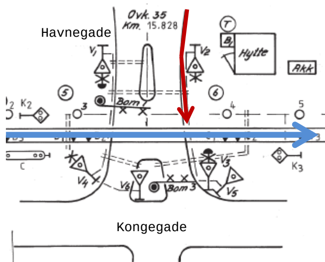
1 Uddrag af kabelplan, overkørsel 35. Rød pil markerer fodgængerens retning ad Havnegade og blå pil marker togets køreretning.
